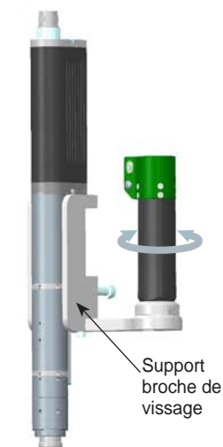
Poignée parallèle à l'axe de vissage, rotative
